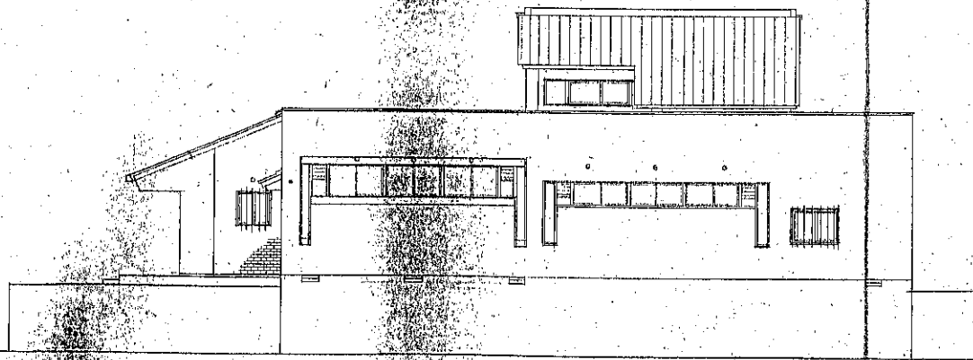
東 立面図 Scale 1:100
