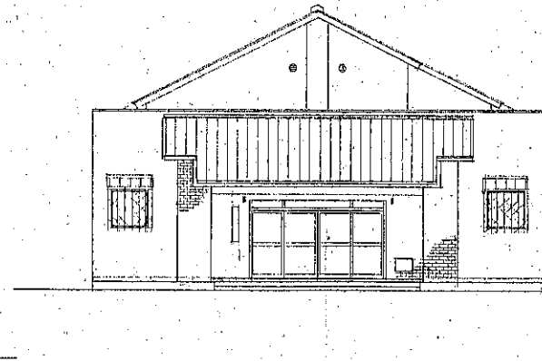
西 立面図 Scale 1:100
