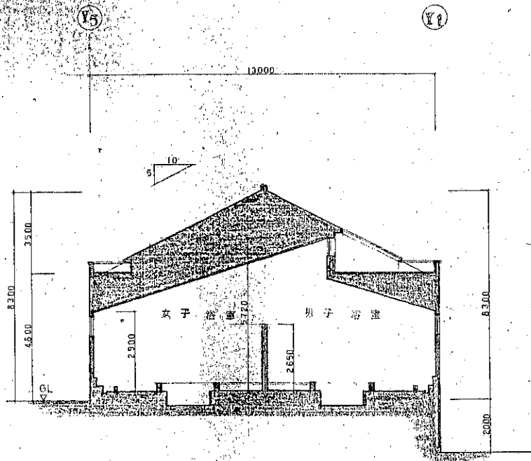
南～北 断面図 Scale 1:100
